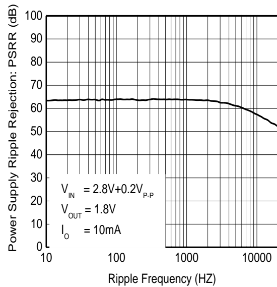
PSRR
