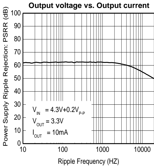
PSRR
